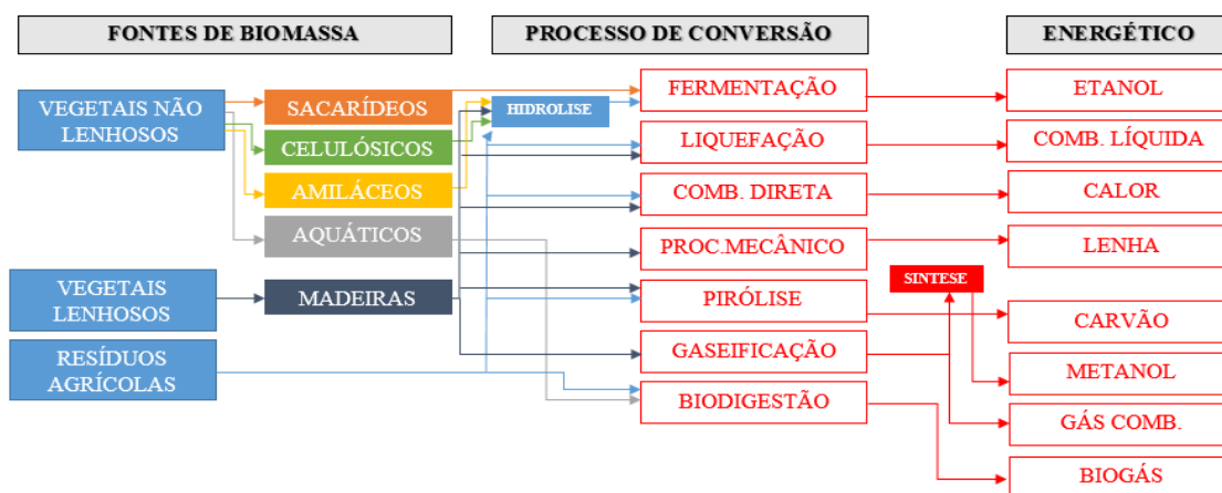
Figura 1 – Diagrama dos processos de conversão energética da biomassa (Fonte: Adaptado de ANEEL, 2010).
